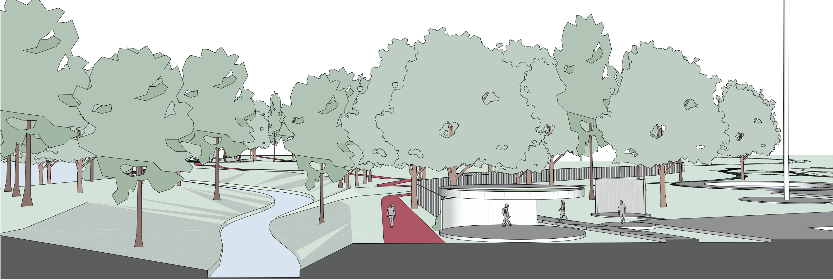
sezione prospettica del collegamento tra Centro Nuoto e il Percorso Natura
